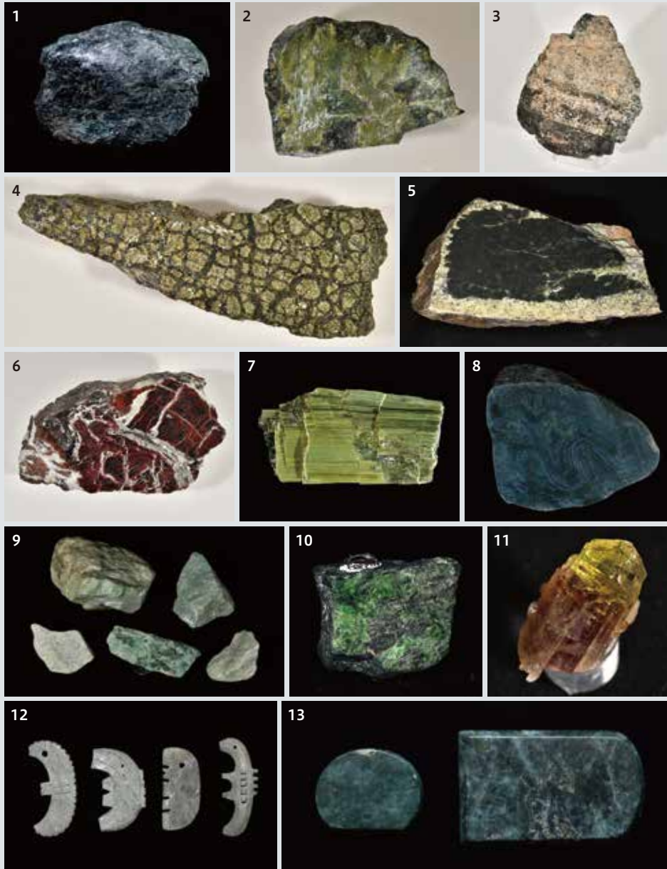
【写真】1. 蛇紋岩 [埼玉県秩父郡皆野町] / 2. オルドビス紀の蛇紋岩 [岩手県遠野市 宮守岩体] (標本提供: 岩手県立博物館) / 3. 蛇紋岩と斑れい岩の接合部 [オマーン] (金沢大学蔵) / 4. 蛇紋岩化作用を受けた直方輝石岩 [トルコ] (金沢大学蔵) / 5. 周辺風化した蛇紋岩 [高知県香美市 白髪岩体] (埼玉大学蔵) / 6. 赤鉄鉱を含む蛇紋岩 [イタリア] (金沢大学蔵) / 7. 繊維状蛇紋石 [群馬県藤岡市 鬼石町 大奈良] (個人蔵) / 8. 軟玉 (ネフライト) [北海道夕張市 白金沢] / 9. 硬玉 (ひすい) の原石 / 10. 灰クロム石榴石 [北海道平取町 日東鉱山] / 11. 蛇紋岩に伴うロディン岩中のベスブ石 [カナダ] (個人蔵) / 12. 滑石製子持勾玉 [行田市北大竹遺跡] (埼玉県教育委員会蔵) / 13. 蛇紋岩製丸轆と蛇尾 [八潮市八條遺跡] (八潮市資料館蔵 / いずれも八潮市指定有形文化財) 【表写真】蛇紋岩 (一面研磨) [埼玉県大里郡寄居町 荒川川原]
